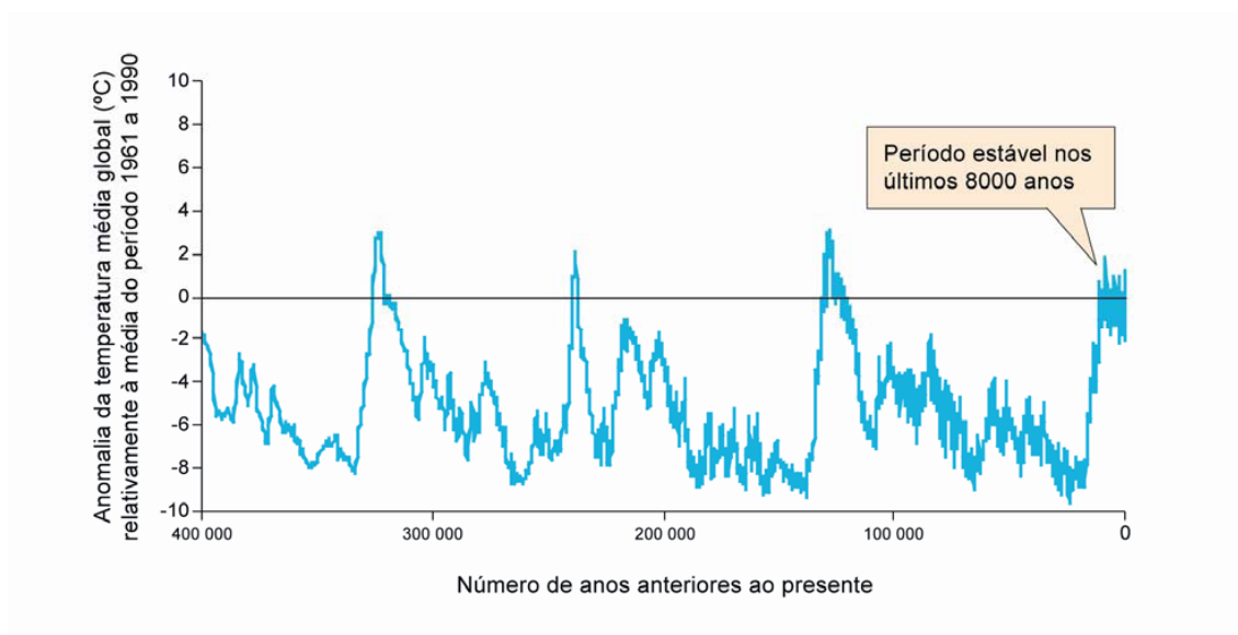
Figura 1: Evolução da temperatura média global da baixa atmosfera, representada por meio da anomalia (diferença na temperatura) relativamente à média do período de 1961 a 1990, nos últimos 400.000 anos.
