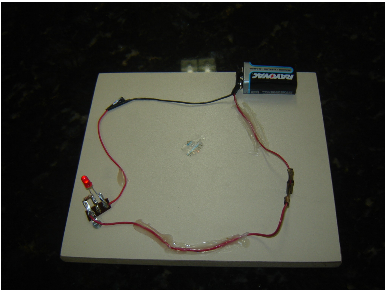
Figura 5 - Circuito elétrico
